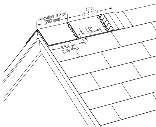
Figure 12-20 : Poser les bardeaux de faîtage en laissant une exposition de 8 po (203 mm) et le fixer avec un clou de chaque côté, de la façon indiquée.
