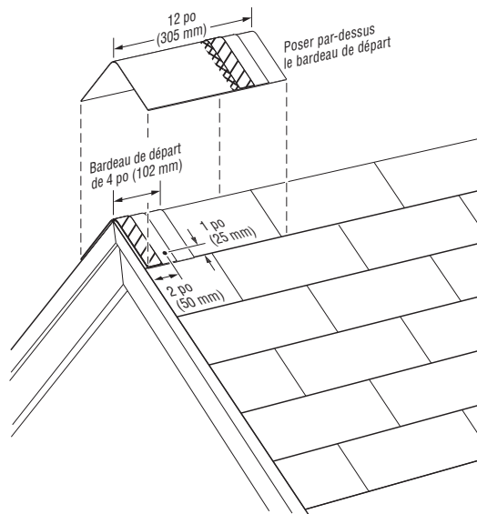
Figure 12-19 : Poser un bardeau de faîtage entier par-dessus le bardeau de départ.
