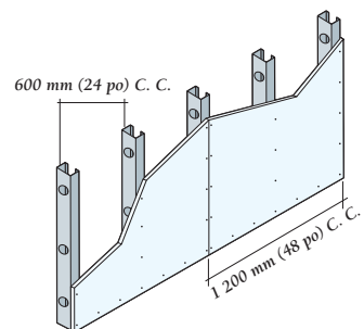
Panneau de revêtement GlasRoc® de type X de 15,9 mm (5/8 po) – Mur à ossature en acier avec espacement des montants de 600 mm (24 po) C. C.
