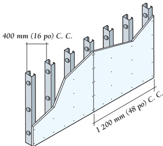
Panneau de revêtement GlasRoc® de 12,7 mm (1/2 po) – Mur à ossature en acier avec espacement des montants de 400 mm (16 po) C. C.
